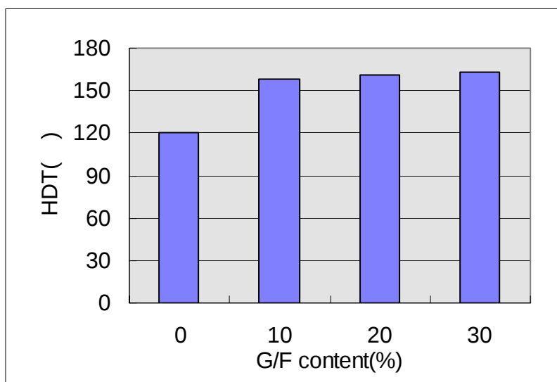
[图2. 玻璃纤维强化时的耐热性]
